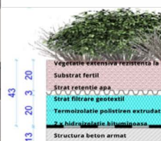
TERASĂ NECIRCULABILĂ
