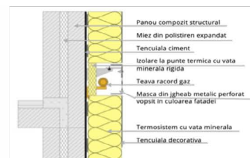
FAȚADĂ
